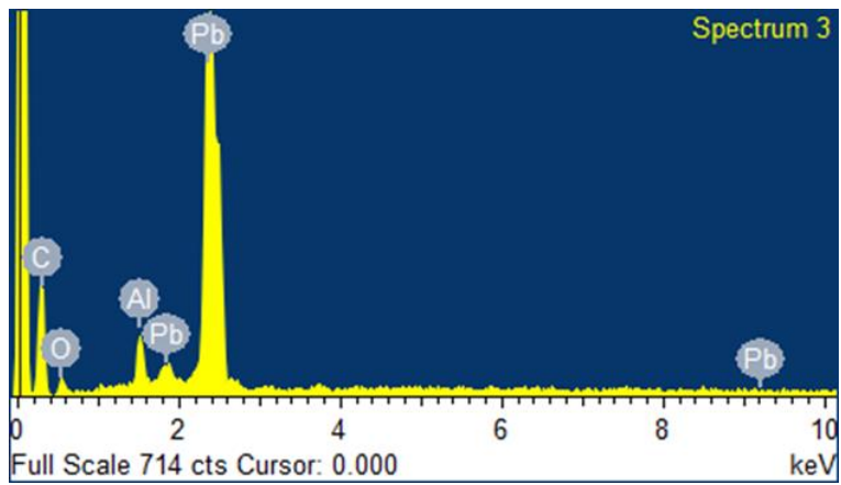
Figura 12. SEM de muestra
