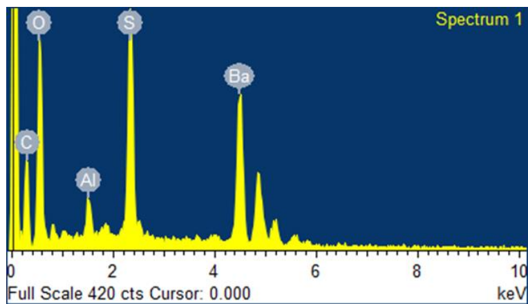
Figura 11. SEM de muestra
