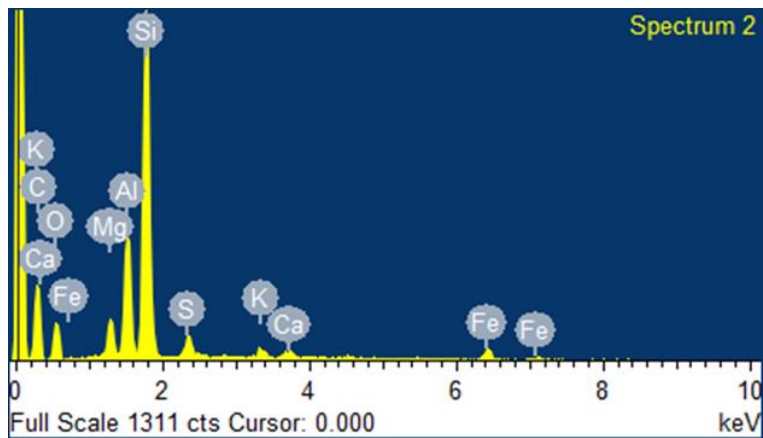
Figura 10. SEM de muestra
