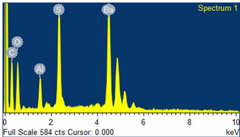
Figura 9. SEM de muestra
