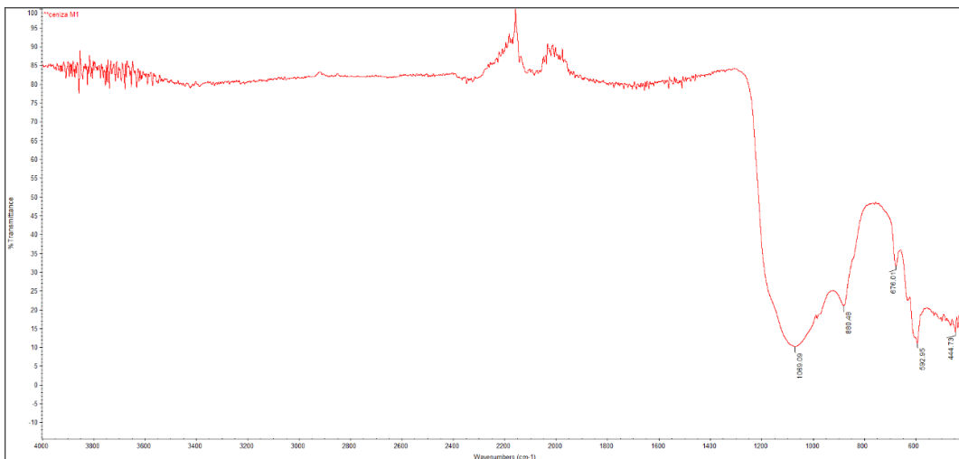
Figura 6. FTIR muestra de ceniza
